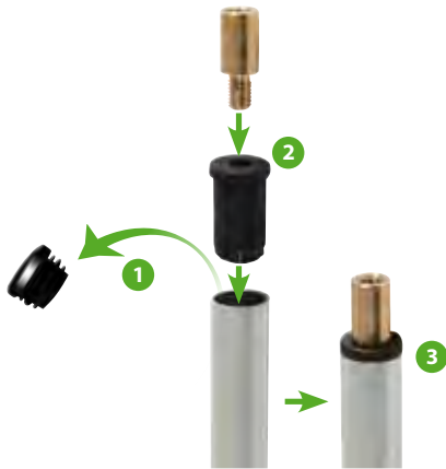
EMBOUT DE PIED TARAUDÉ POUR ACCESSOIRES Foot tip accessories
